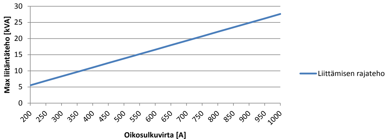
Kuva 2. Tuotantolaitoksen maksimi liittämäteho liityntäpisteen oikosulkuvirran funktiona.
